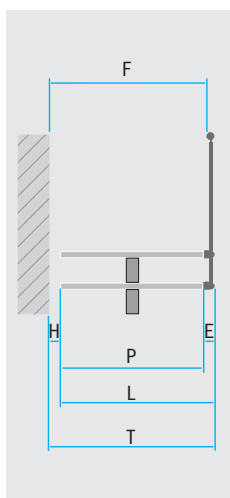
näkymä edestä yksipuolisella kaiteella
