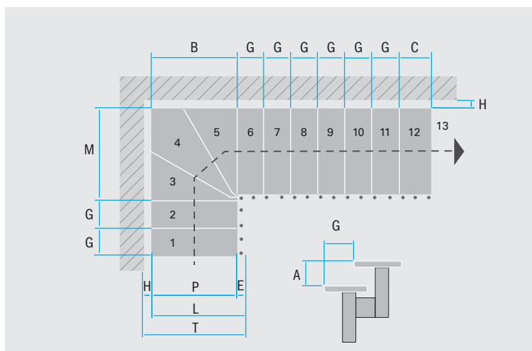
tasonäkymä ja mitat
